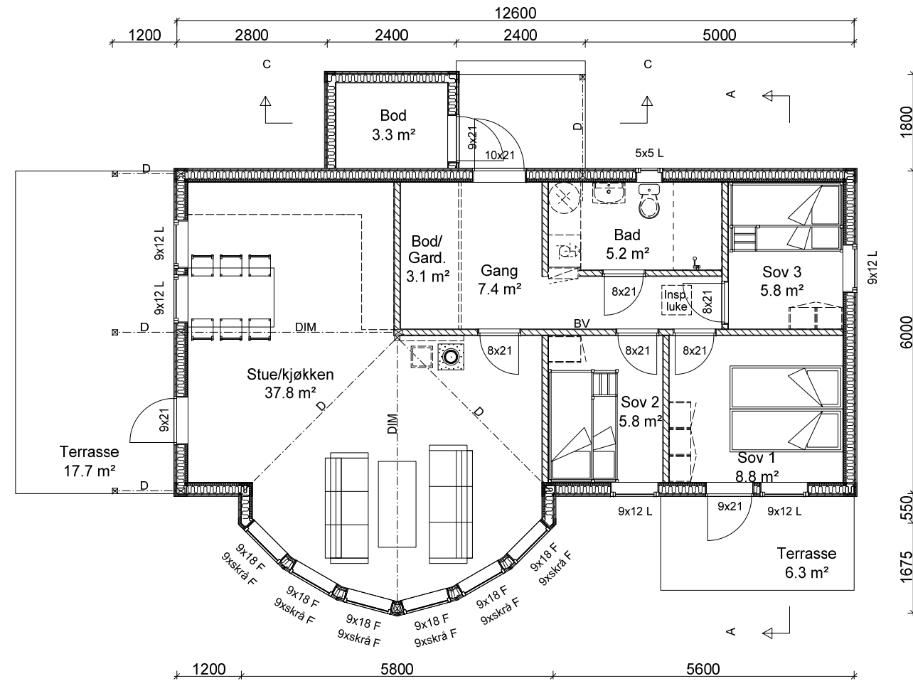
PLAN 1.ETASJE
