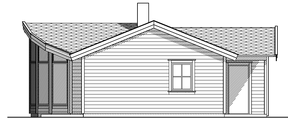
FASADE MOT
