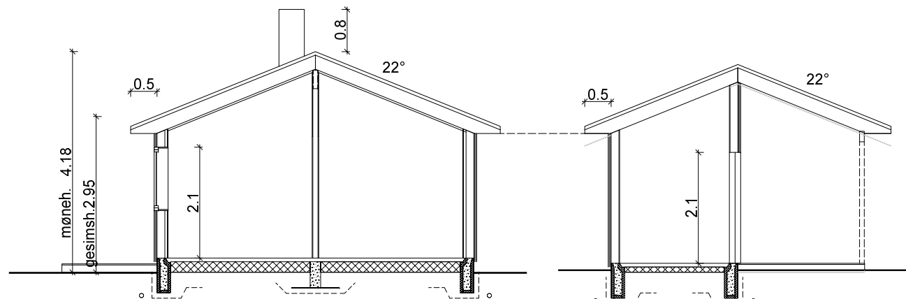
SNITT A-A
