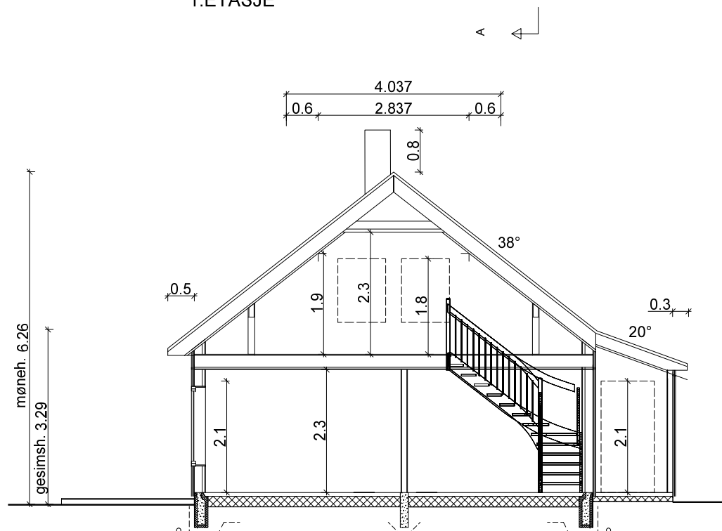
SNITT A-A
