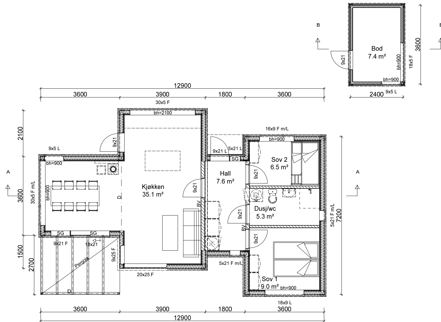
PLAN 1 ETG.
