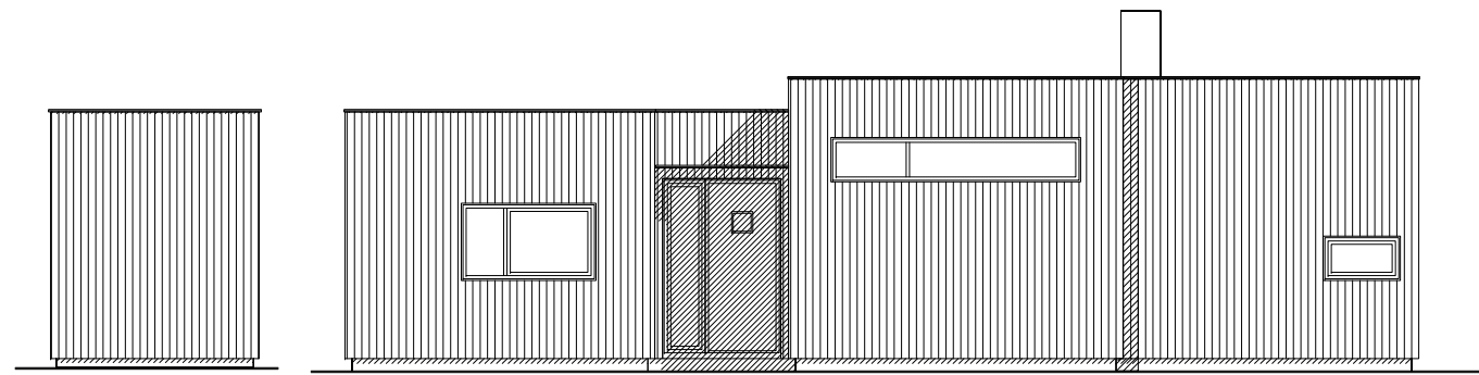
FASADE MOT
