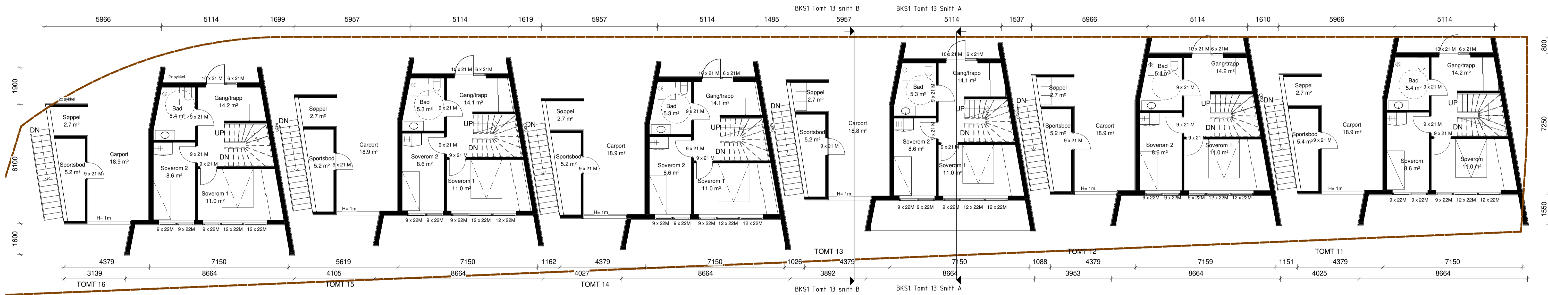
BKS1 Plan 1 1 : 100
