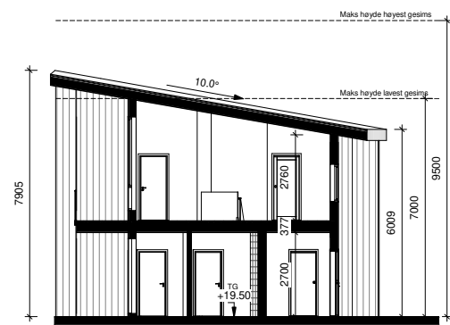
BKS4 Bolig A 1 : 100
