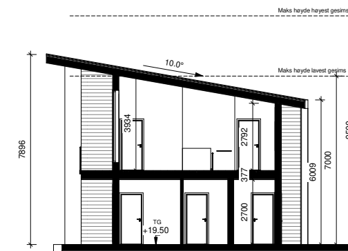
BKS4 Bolig B 1 : 100
